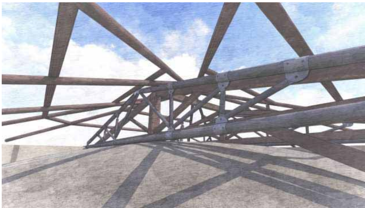
Ricostruzione tridimensionale di progetto per la nuova struttura di copertura della cupola della Chiesa Parrocchiale.
